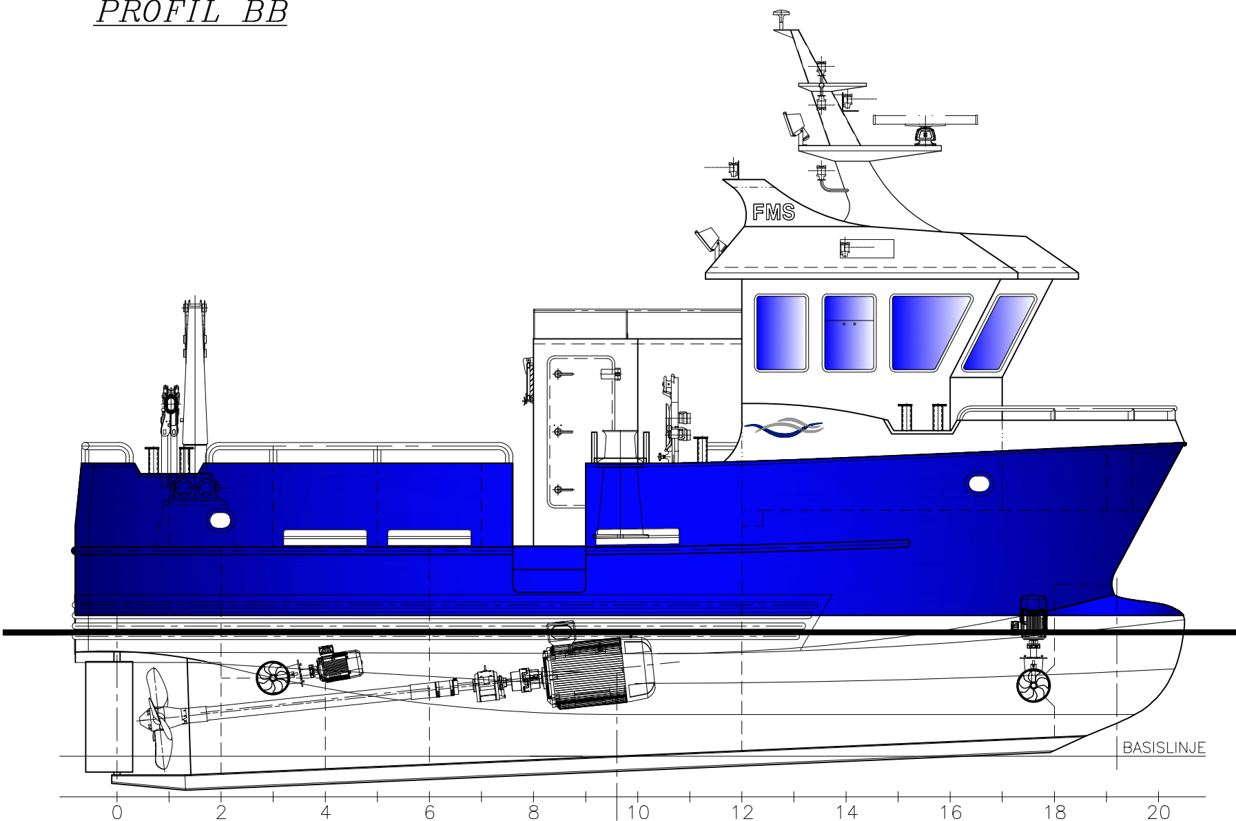
PROFIL
