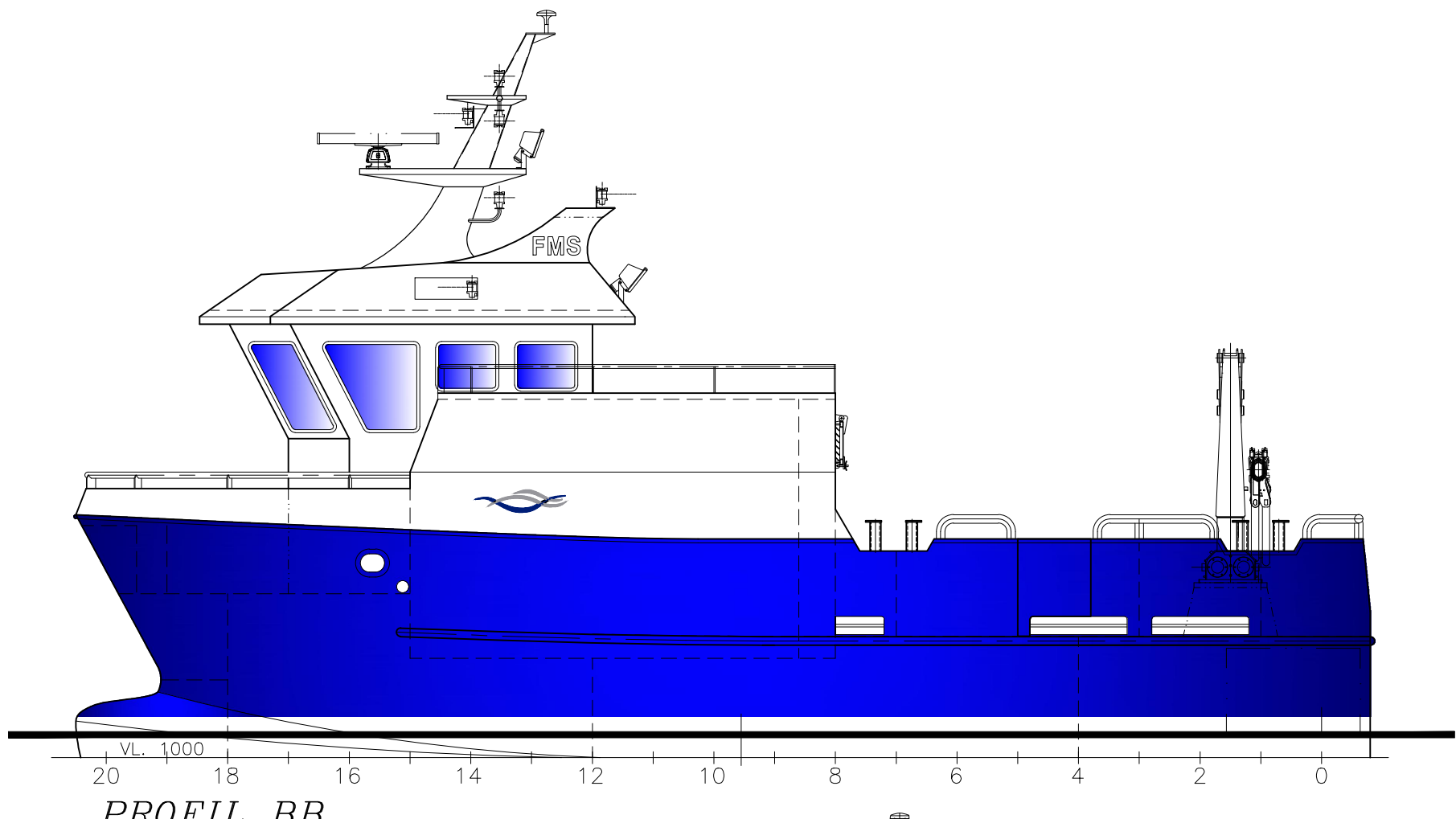
PROFIL BB
