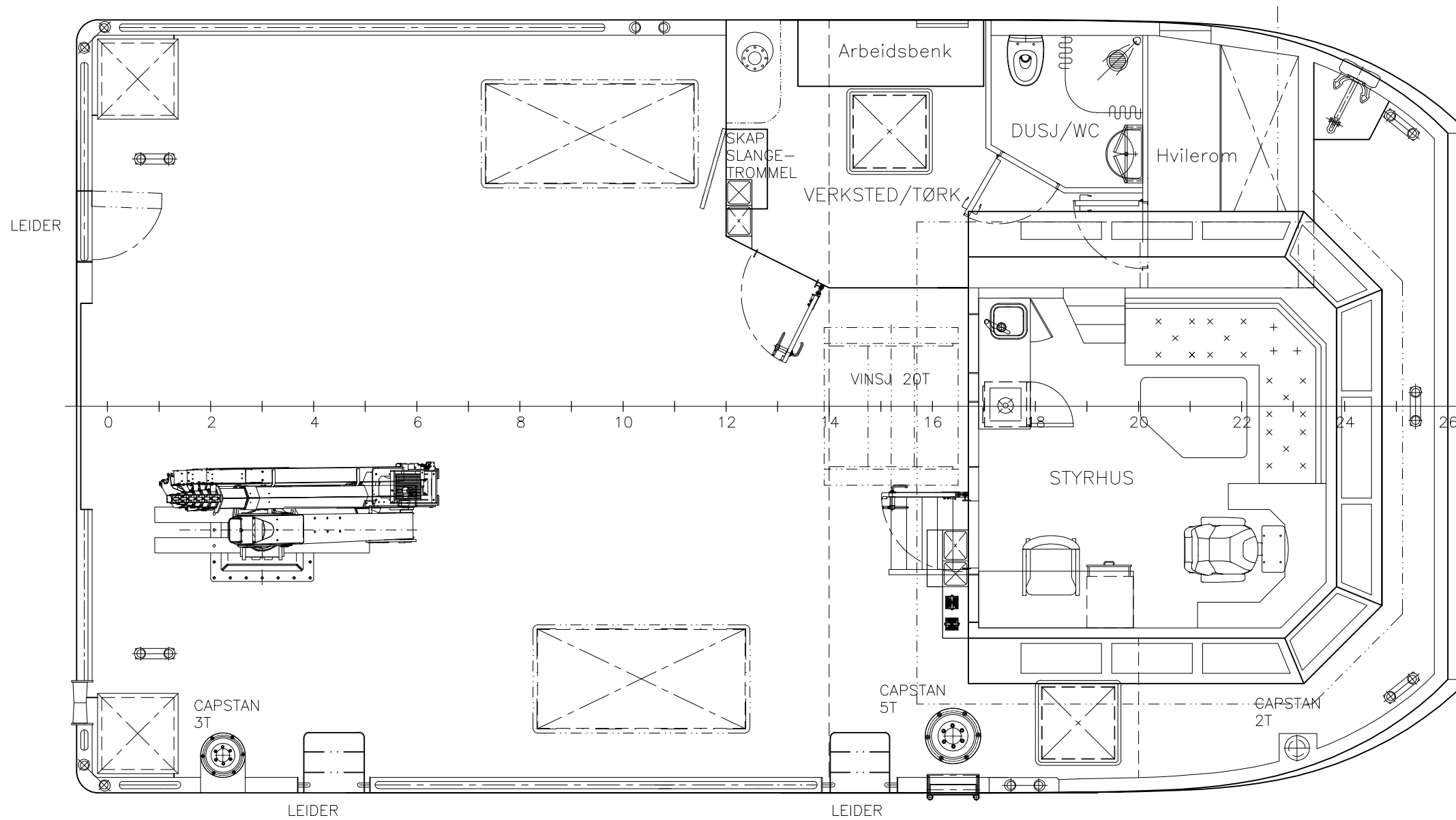
HOVEDDEKK
