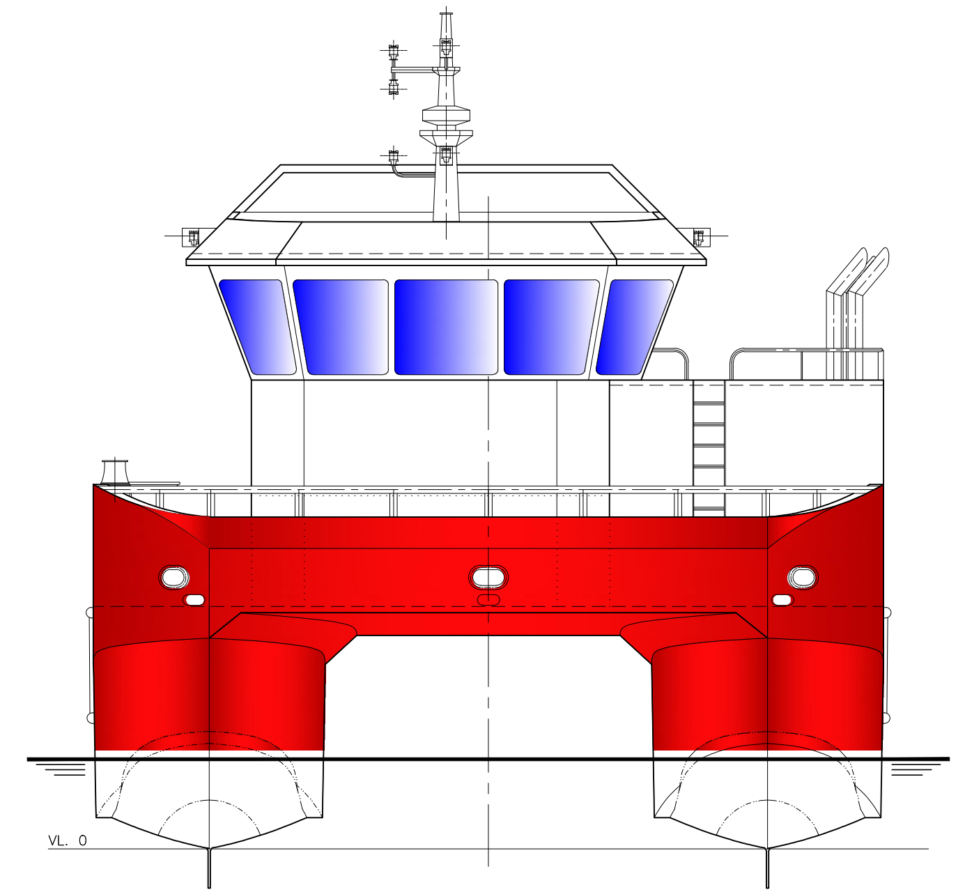
SETT FORFRA
