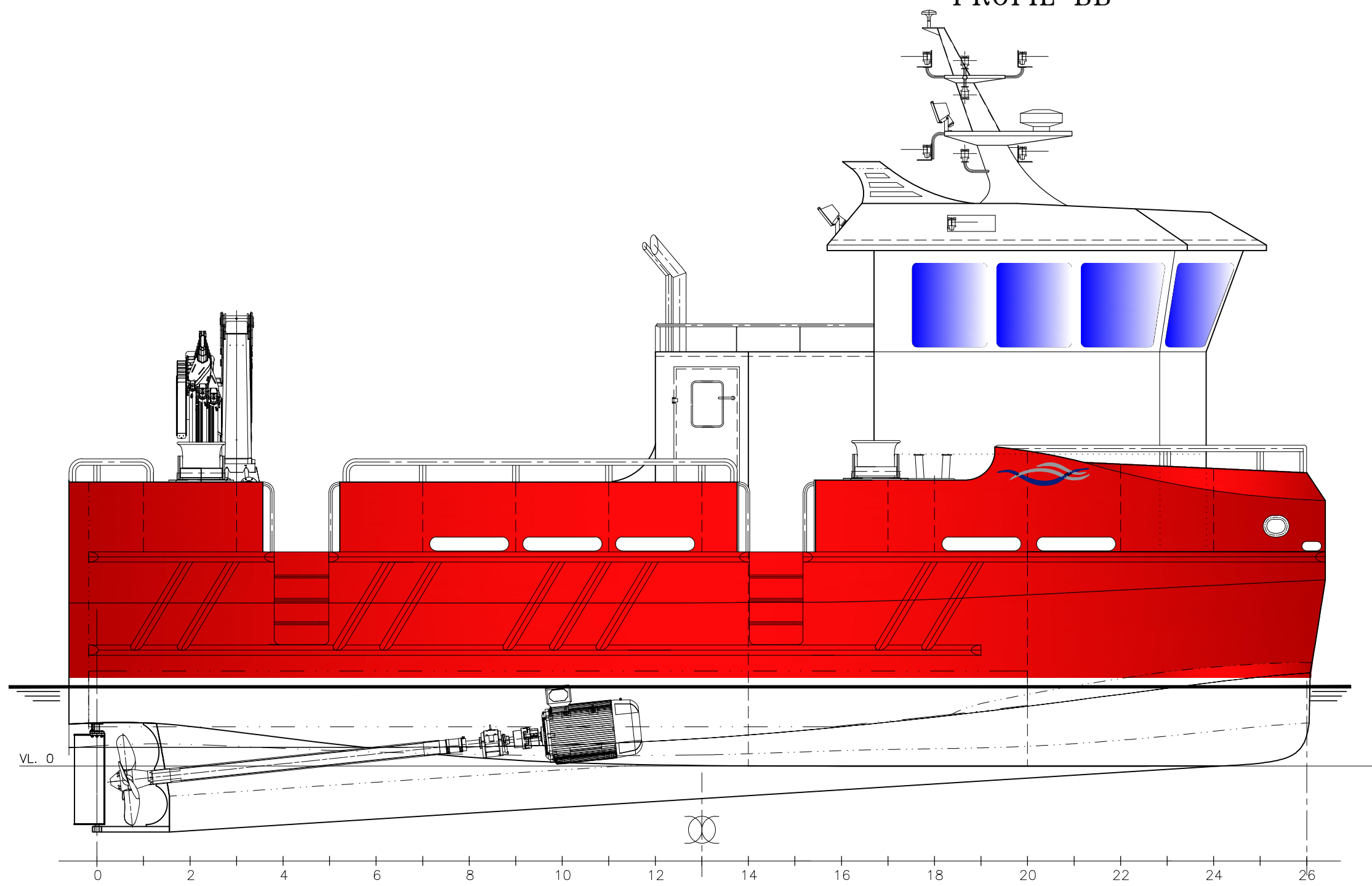
PROFIL SB
