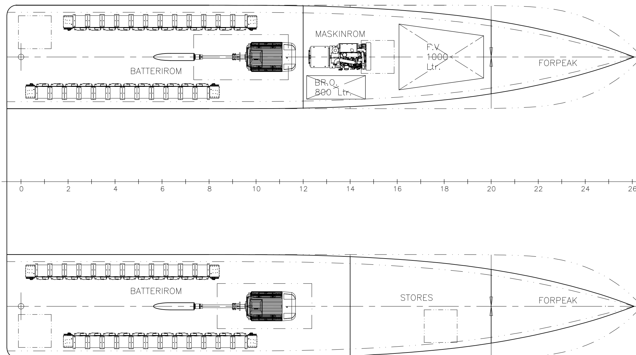
UNDER HOVEDDEKK
