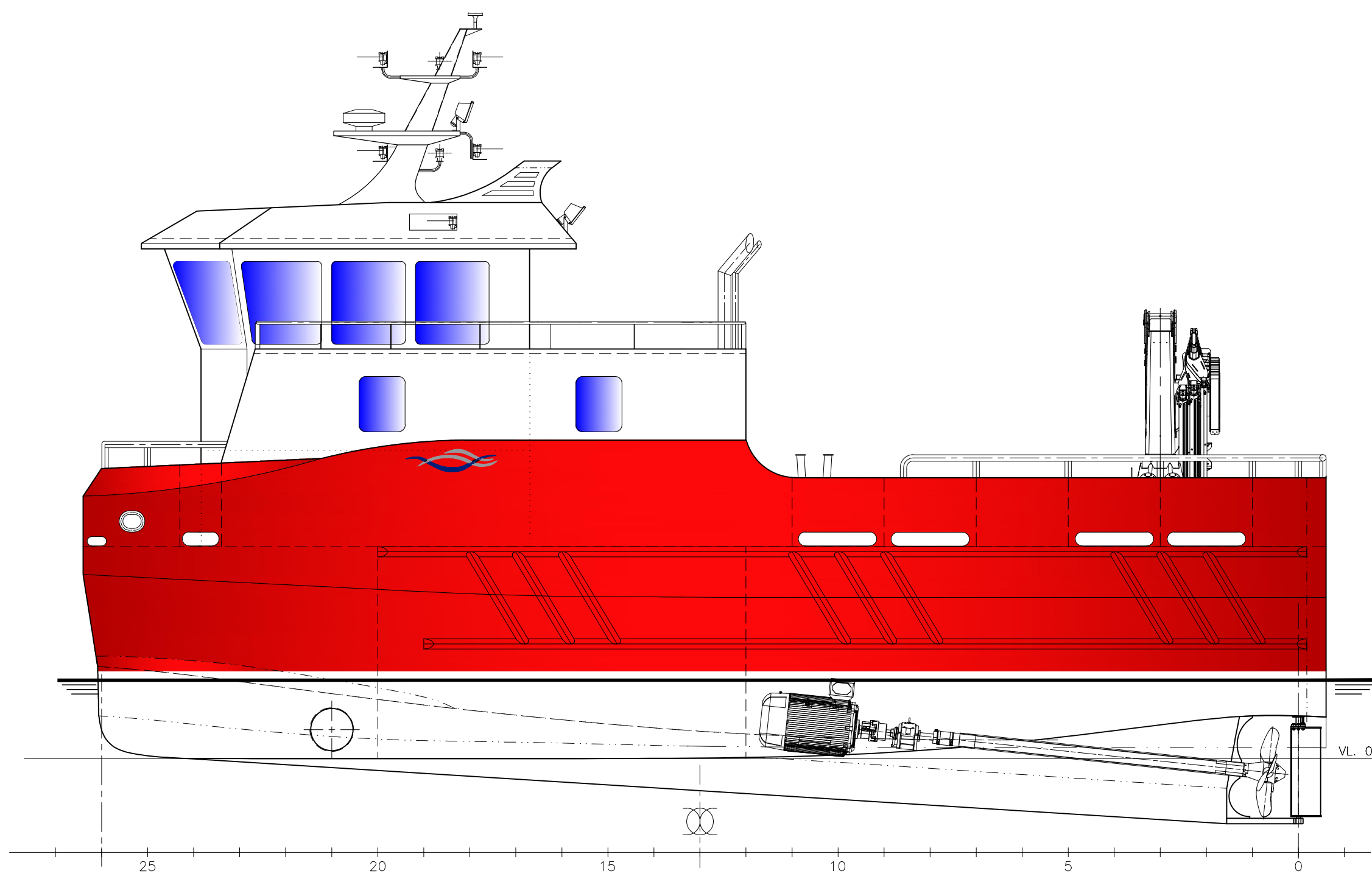
PROFIL BB
