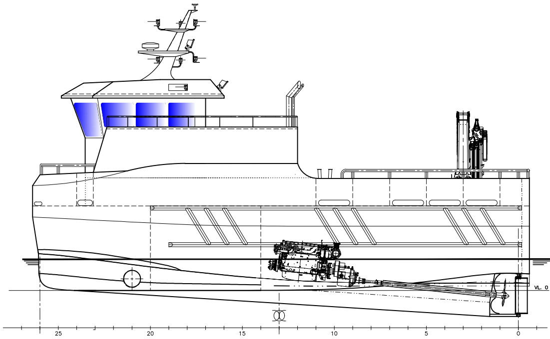
PROFIL BB
