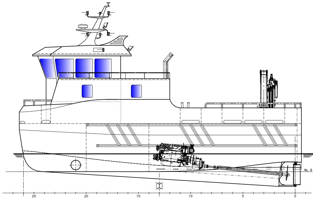
PROFIL BB
